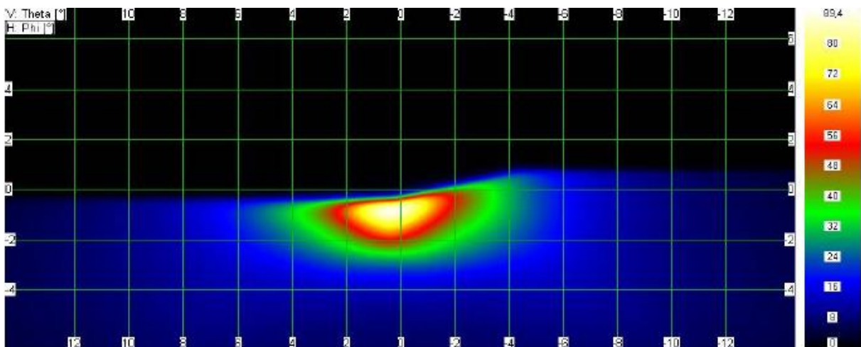
光强分布图
